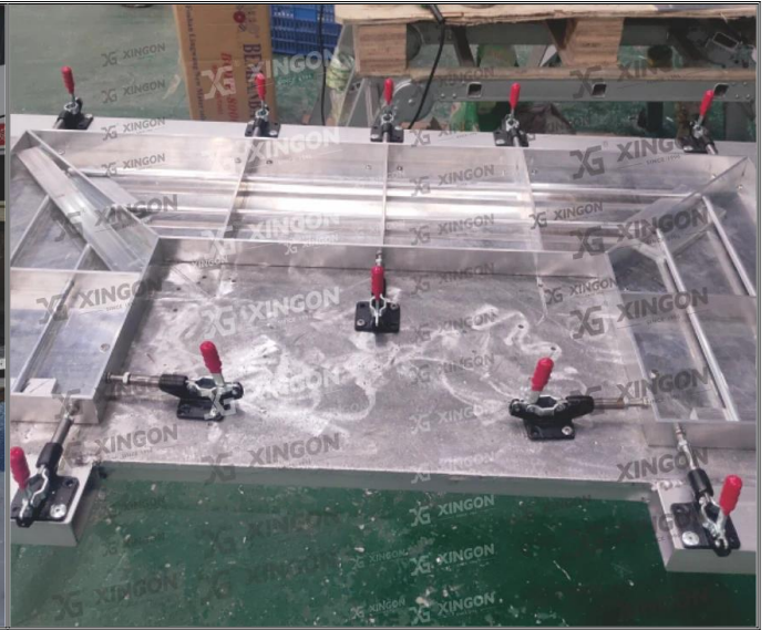
Profilbefestigung - Schweißen
